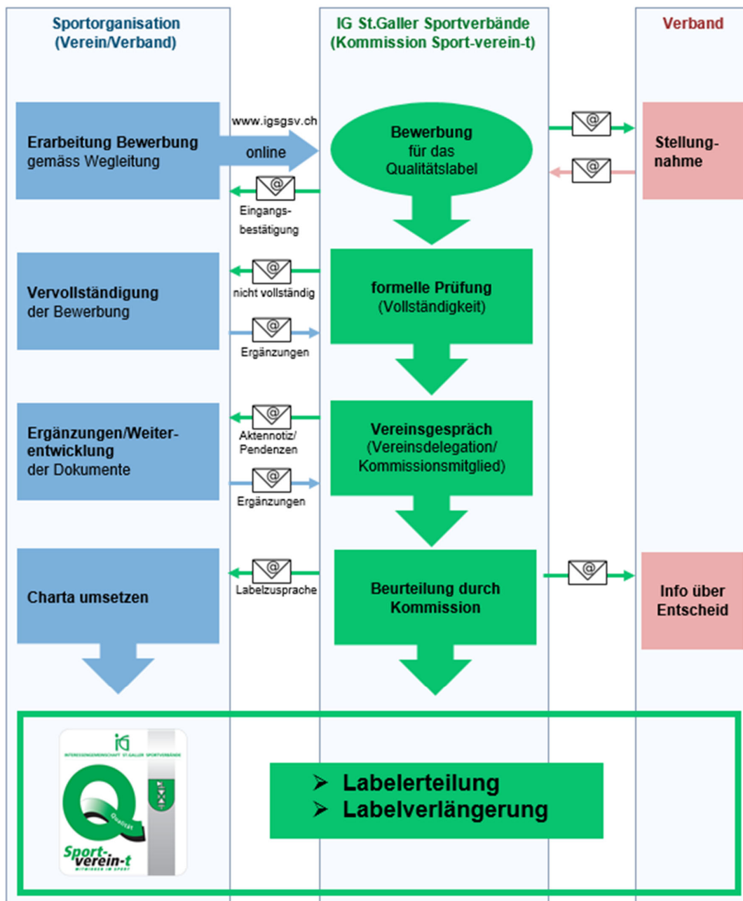
Abbildung 2: Bewerbungsprozess Sport-verein-t.
